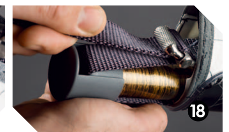
VARIO TOP Le Vario Top permet d'ajuster votre voile en fonction de la taille de votre mât. L'ajustement de longueur s'effectue grâce à la sangle de réglage et le capuchon de têtère.
