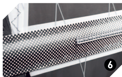
POCKET GUARD Une protection PVC transparente vient protéger le fourreau de la première latte sur toute sa longueur contre tout frottement.
